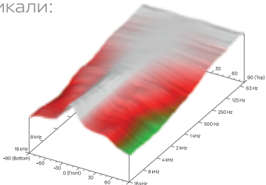
Диаграмма направленности C30
