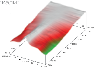
Диаграмма направленности H30
