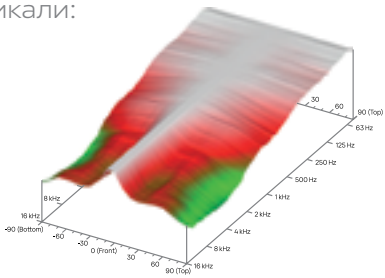
Диаграмма направленности H10
