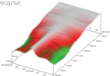
Диаграмма направленности C10
